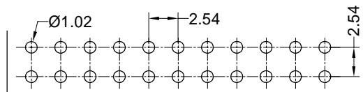
P.C.B LAYOUT
